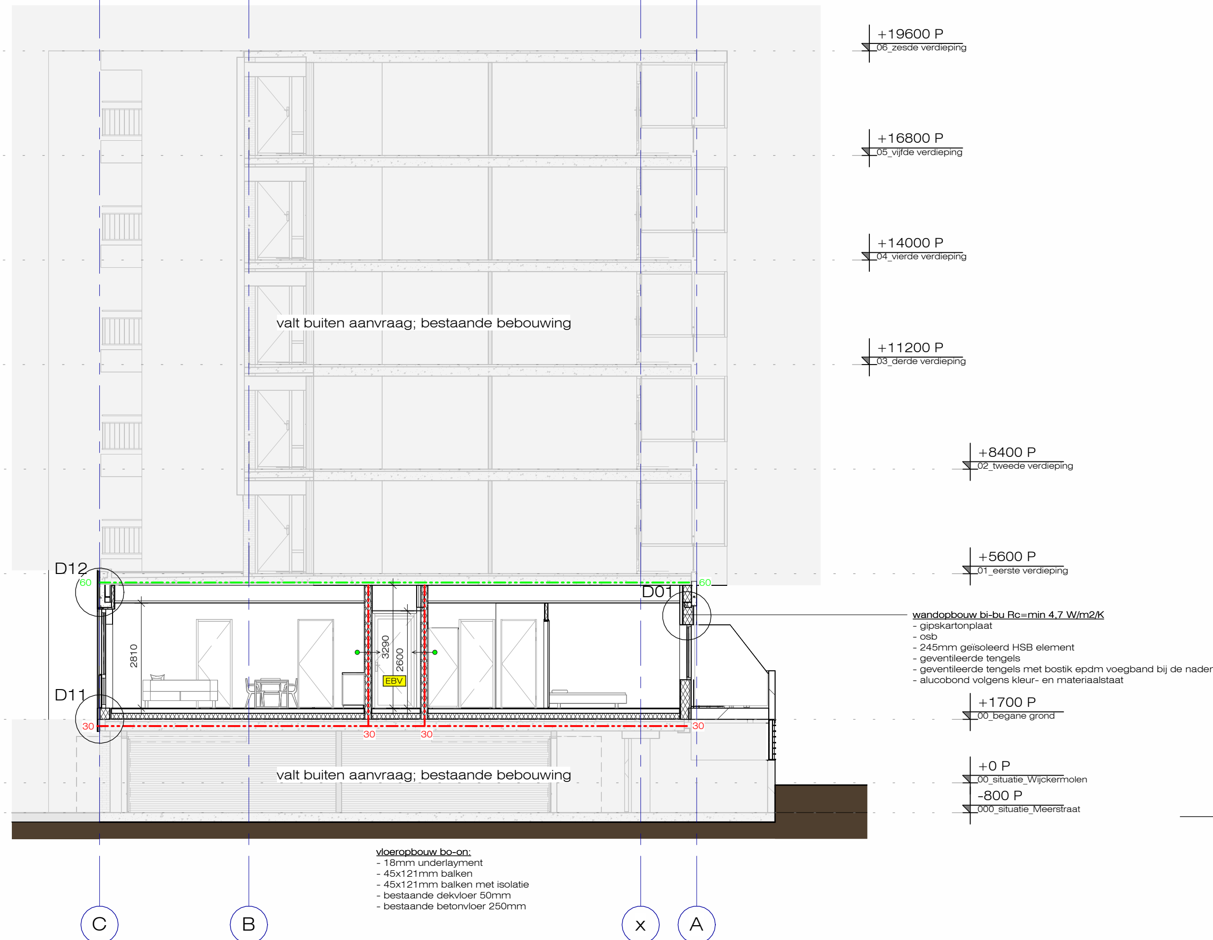
DO Doorsnede AA
