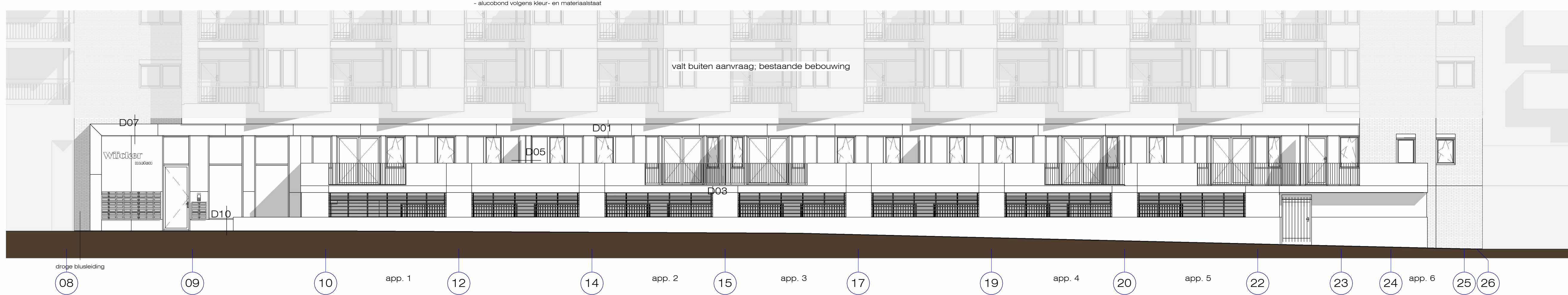
201-DO Zuidgevel
